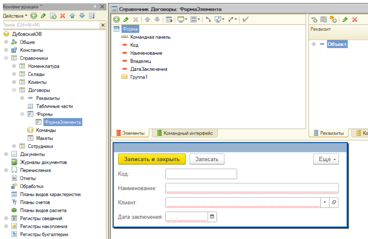
Рисунок 3 – Готовая форма
