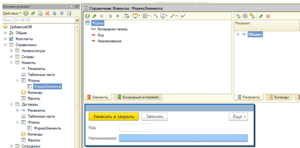
Рисунок 4 – Справочник Клиенты
